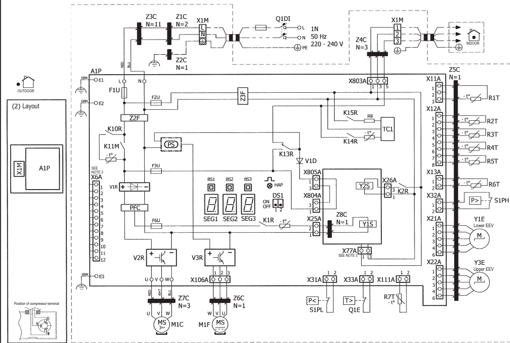
AZAS71MV1, RZASG71MV1
